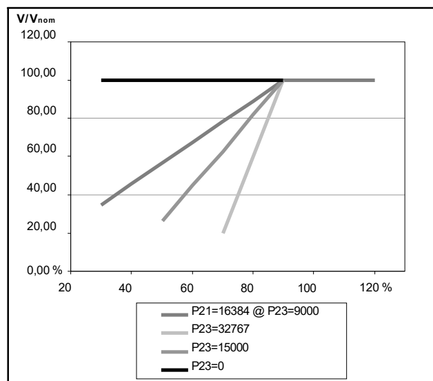
Abb. 10 b: Einstellung der V/F-Steigung, P[23]
