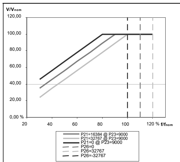
Abb. 10 a: Unter- und Überdrehzahl, P[21] und P[26]
